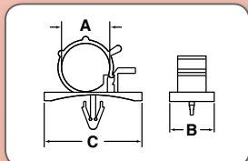
CCP Pino de Encaixe
